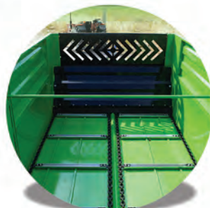
Doppelreihiges Kettenfördersystem Double row chain conveyor system
