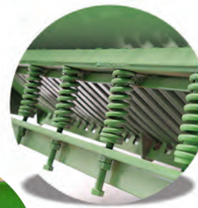
Siebsystem mit Feder Screen system with spring
